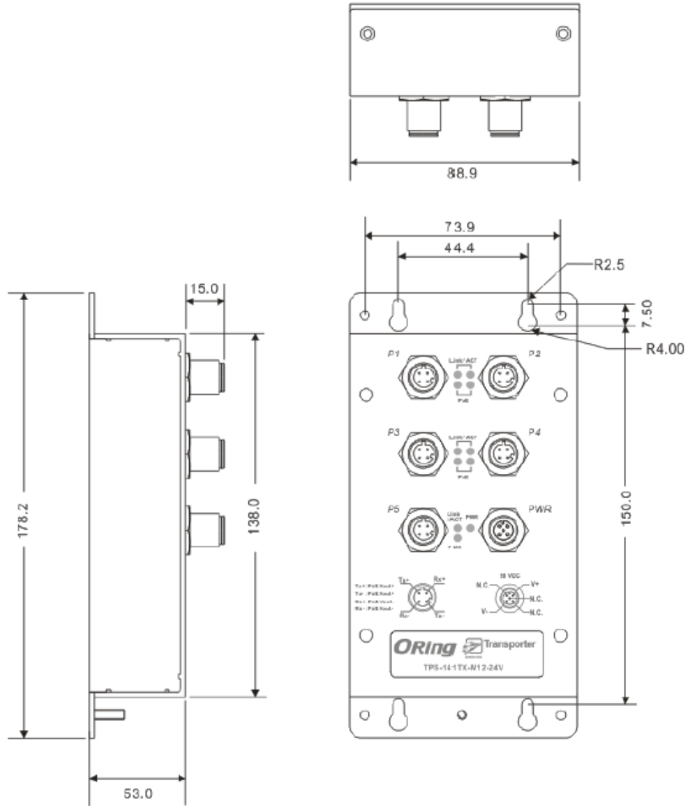
TPS-141TX-M12-24V/MV
