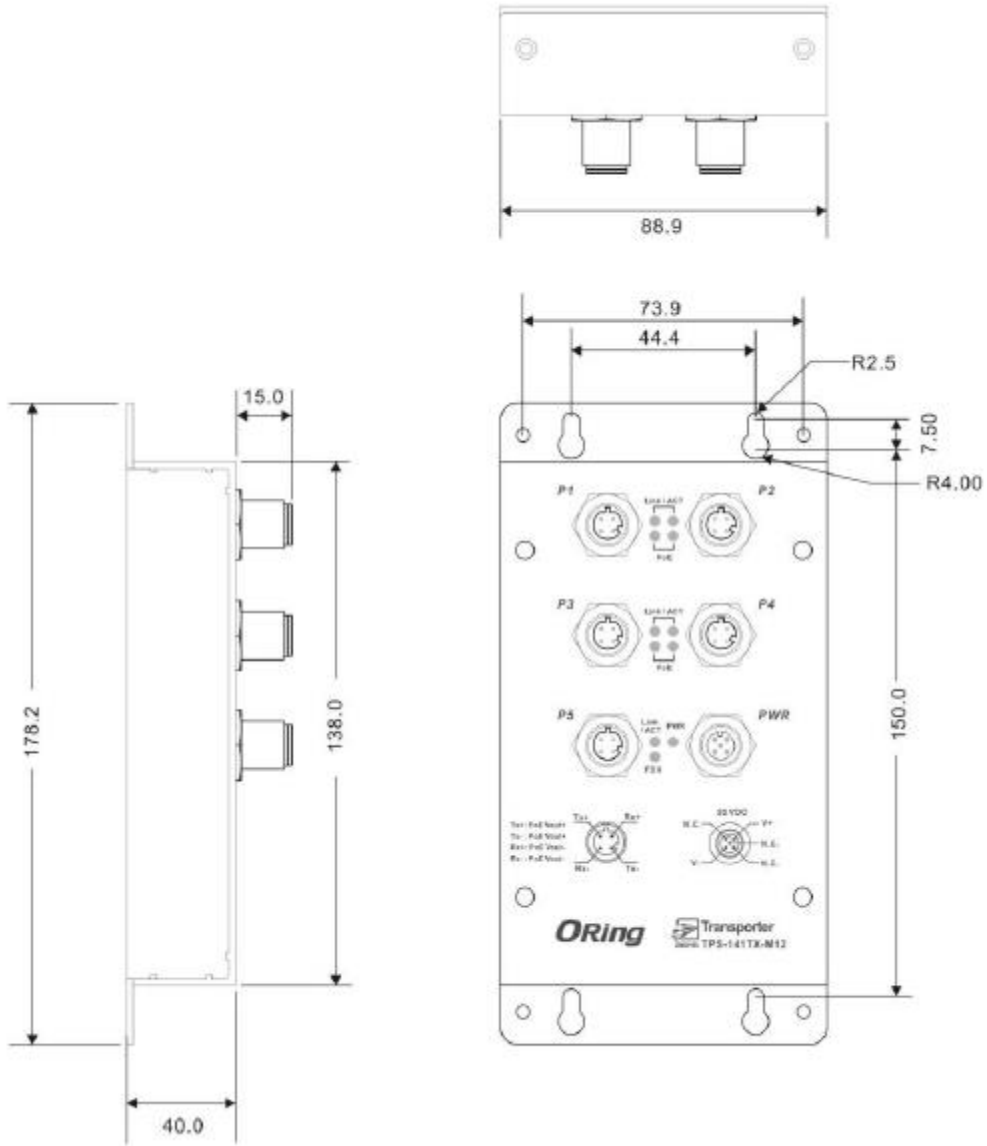
TPS-141TX-M12
